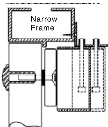
Narrow door frame(swing out)
