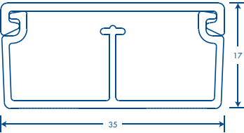
Esquinero exterior
