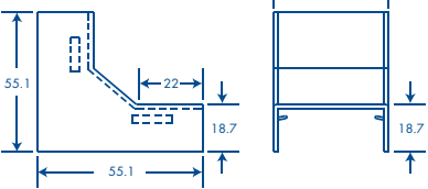
Esquinero interior
