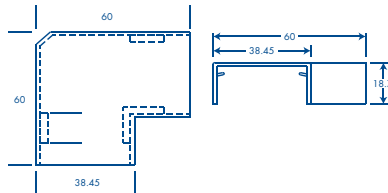
Sección T
