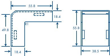
Esquinero interior
