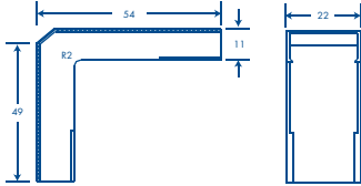
Esquinero interior
