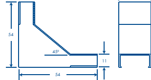
Pieza unión
